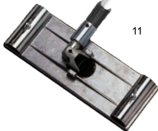
11 Stielschleifer Metal-Teleskop. Für Schleifgitter (Nr. 4). Mit Klemmleisten,
